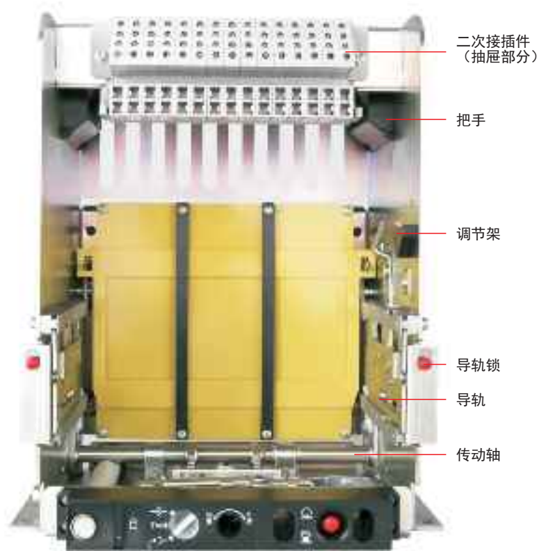
HYW3-1600/3抽屉座
