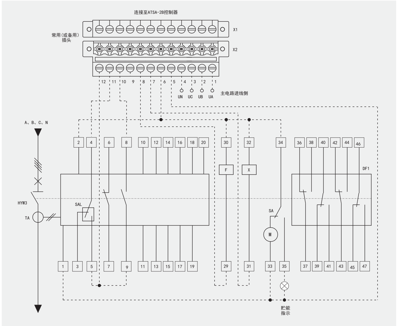
双电源控制器接线图
