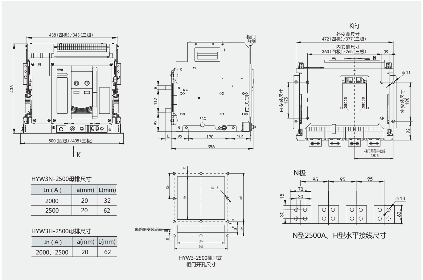
HYW3-2500抽屉式外形及安装尺寸(内安装尺寸或外安装尺寸只选其中一种进行固定)
