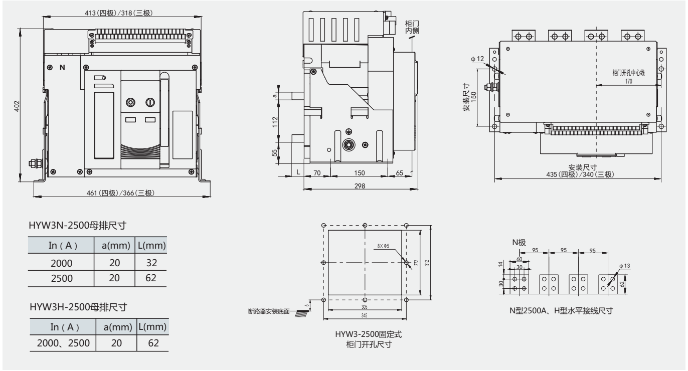
HYW3-2500抽屉式外形及安装尺寸(内安装尺寸或外安装尺寸只选其中一种进行固定)
