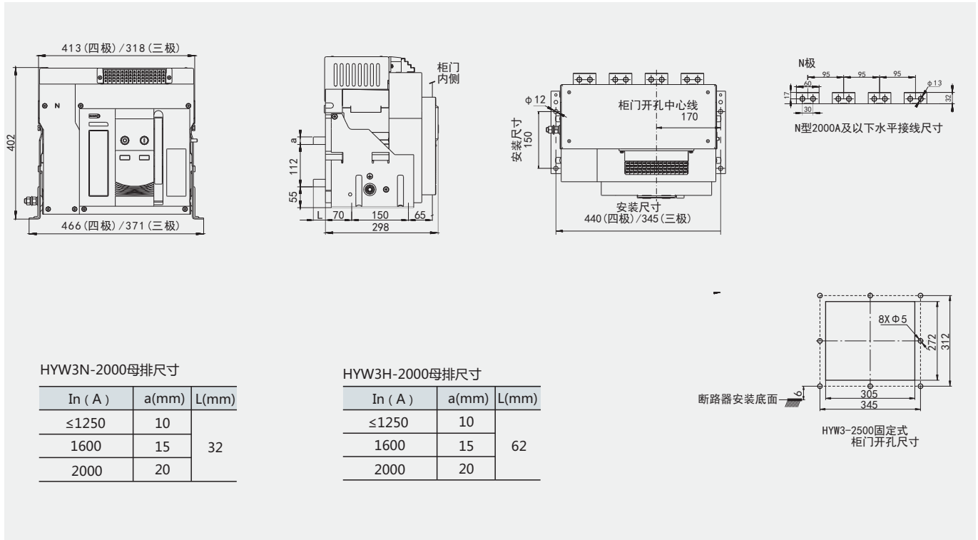
HYW3-2000固定式外形及安装尺寸
