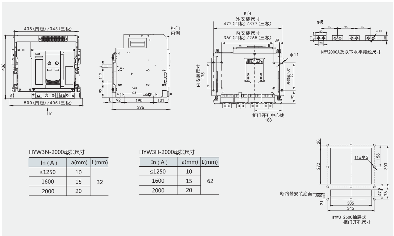
HYW3-2000抽屉式外形及安装尺寸(内安装尺寸或外安装尺寸只选其中一种进行固定)
