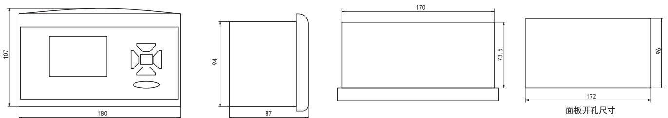
双电源控制器外形及安装尺寸
