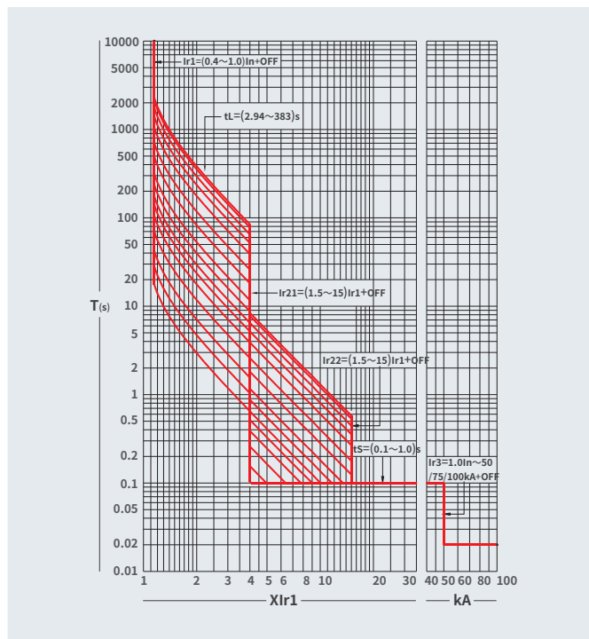
图 4、特快反时限（马达保护）
